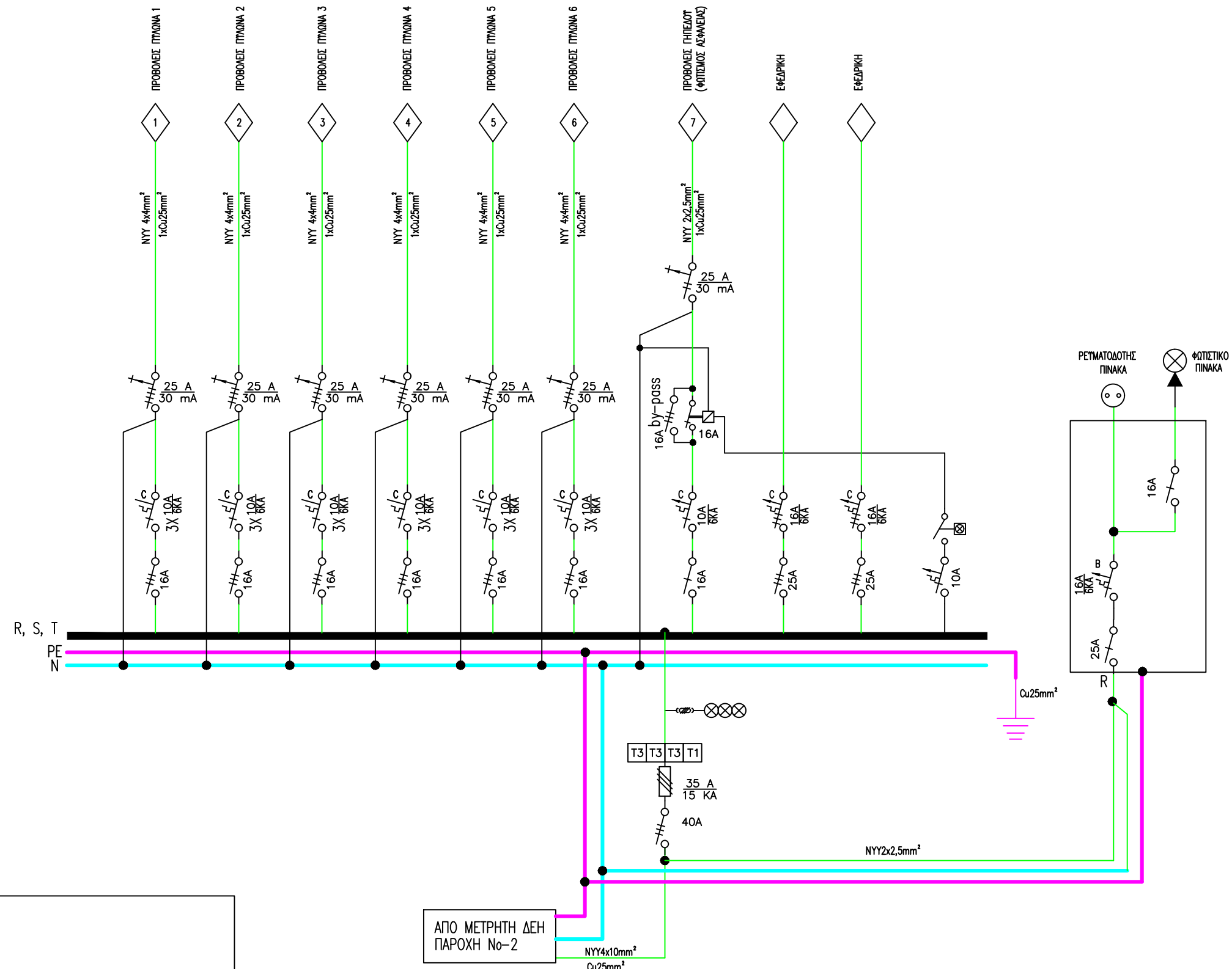
ΔΙΑΓΡΑΜΜΑ ΗΛΕΚΤΡΙΚΟΥ ΠΙΝΑΚΑ
