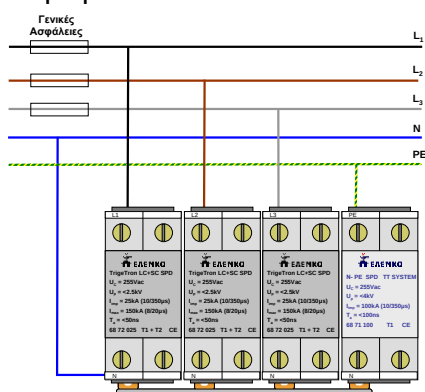
Εικόνα 1: Εγκατάσταση μονοπολικών απαγωγών πρωτεύουσας και δευτερεύουσας προστασίας (T1+T3) σε τριφασικό σύστημα για συστήματα σύνδεσης γειώσεων TN και TT
