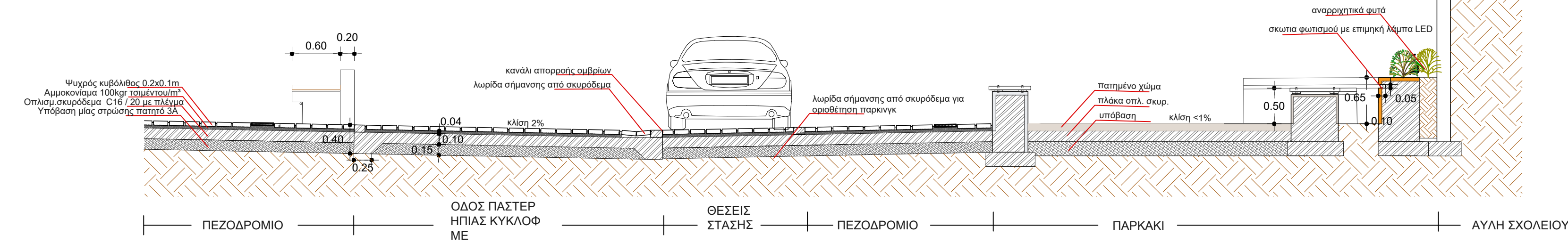
TOMH 4-4 1:50
