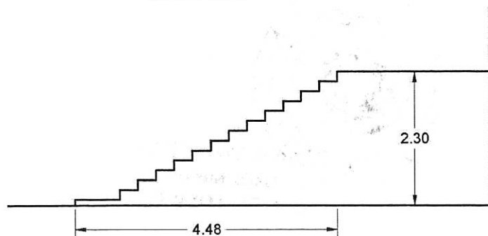
ΤΟΜΗ
