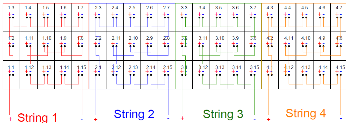
Εικόνα 3 Ενδεικτική διάταξη φωτοβολταϊκών πλαισίων και στοιχειοσειρών για στέγαστρο 8 θέσεων.
