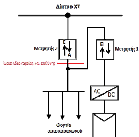
Εικόνα 1 Τυπικό σχήμα σύνδεσης ΦΒ συστήματος αυτοπαραγωγής σε εγκατάσταση Χρήστη του Δικτύου ΧΤ
